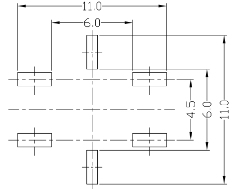
P.C.B. LAYOUT
