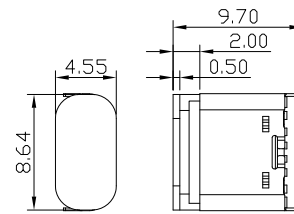
加塞子不盖图 SCALE 2:1
